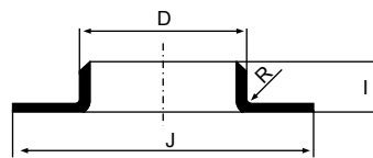
PESTANA ESTAMPADA
