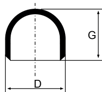
CAP
